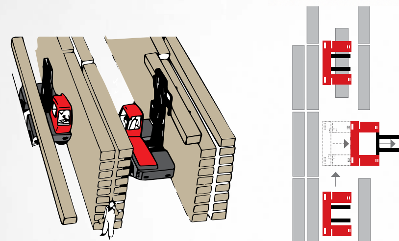
Wózek boczny typu Sideloader: Optymalne wykorzystanie przestrzeni
